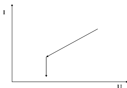
图 4.6 定电阻转换定电压模式
