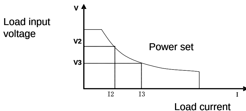
图 4.9 定功率模式
