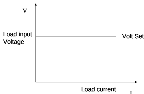
图 4.7 定电压模式
