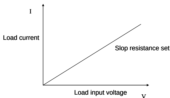
图4.5 定电阻模式
