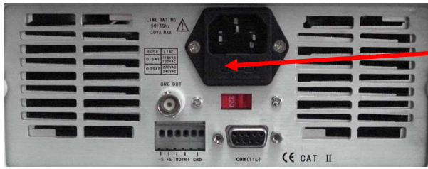
图3.1 保险丝位置
