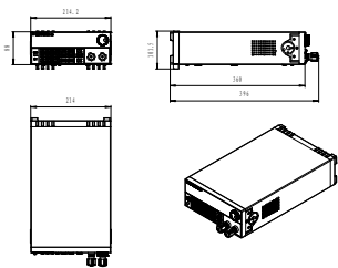
2U（窄）仪器（无橡胶套和把手）外形结构示意图
