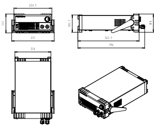
2U（窄）仪器外形结构示意图
