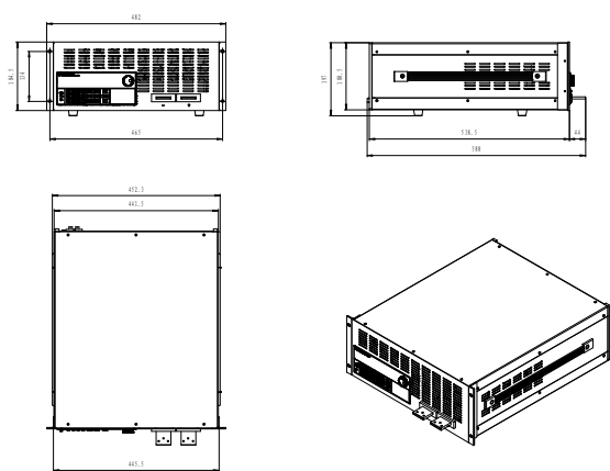
4U（480A）仪器外形结构示意图
