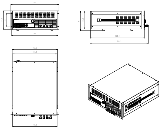
4U（250A）仪器外形结构示意图
