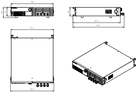
2U（宽）仪器外形结构示意图
