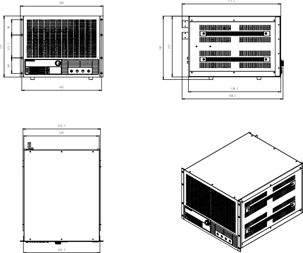
8U仪器外形结构示意图
