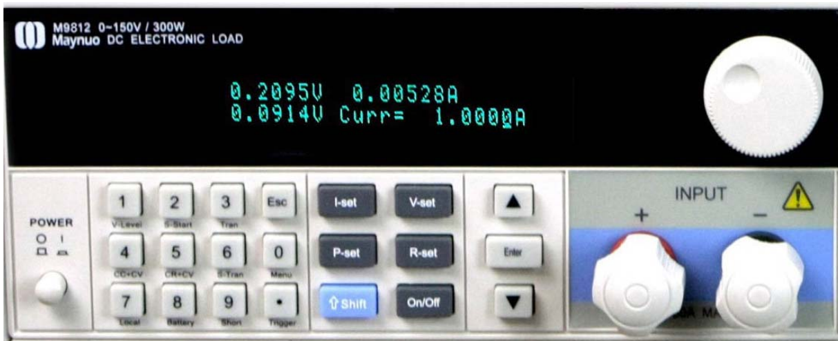
图3.2 前面板图
